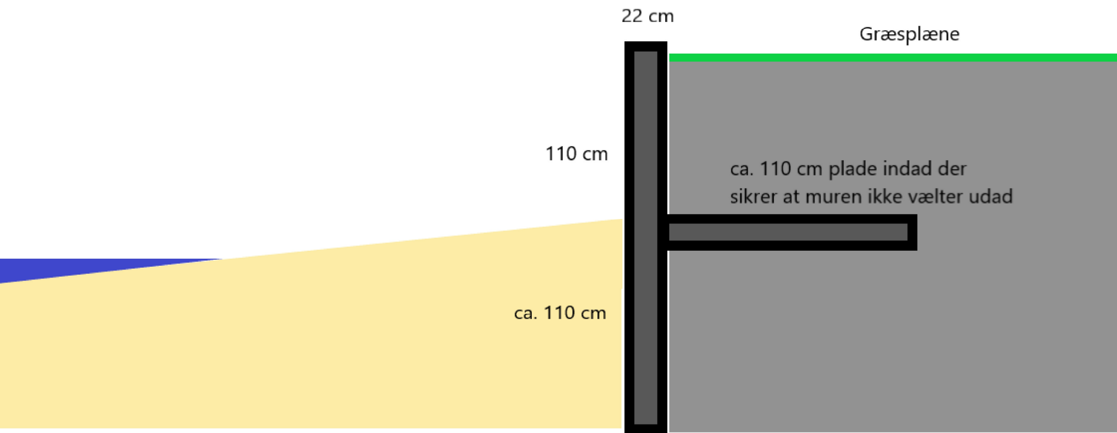
Profil som eksisterende mur
